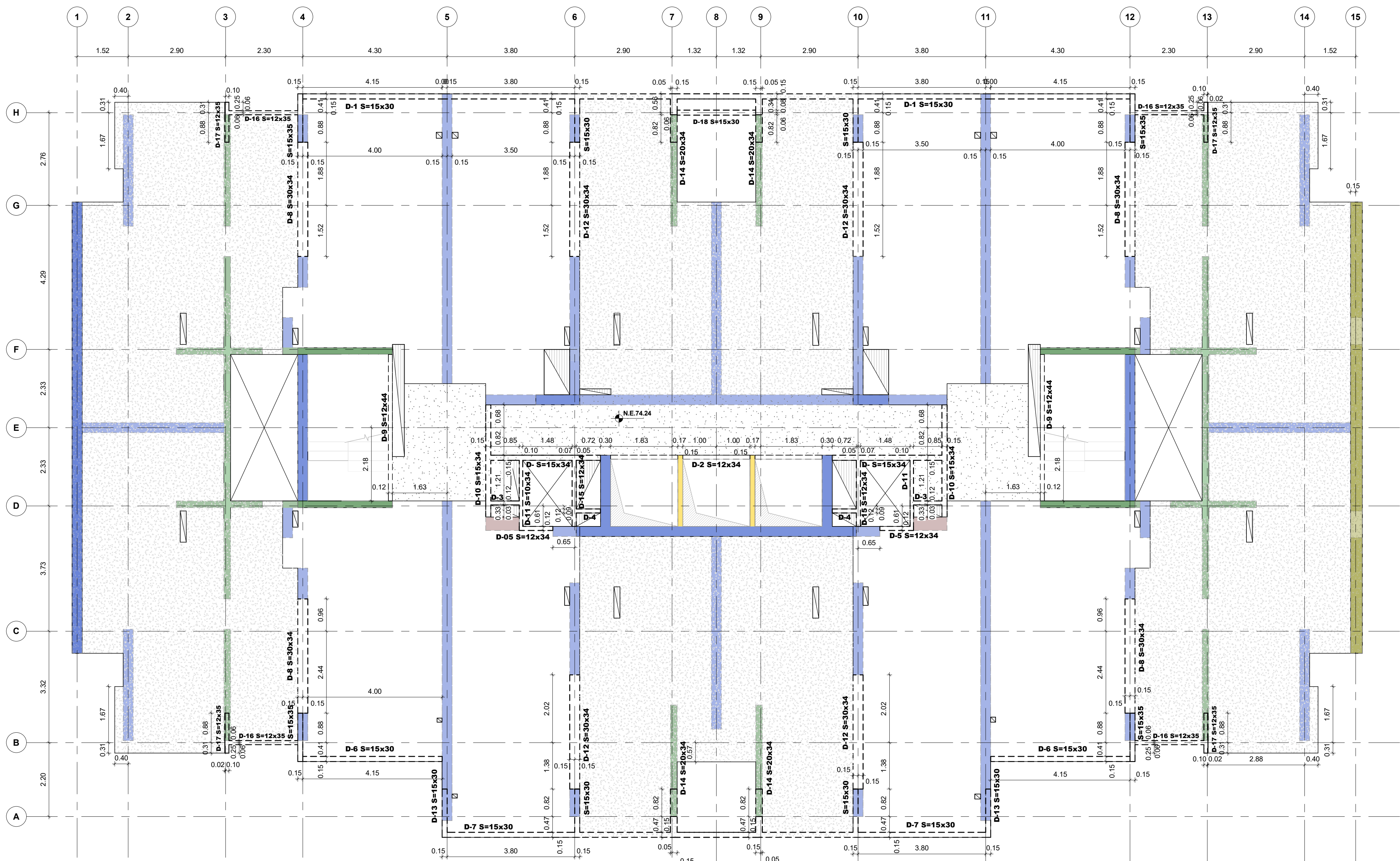
PLANTA LOCALIZACIÓN DE DINTELES CUBIERTA Escala 1 : 75
